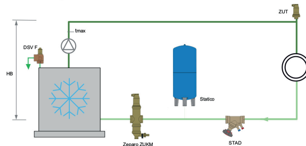
Køleanlæg
