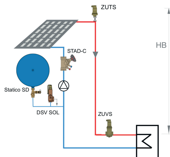
Solvarme
